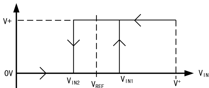
图2 非反向迟滞比较器电路
